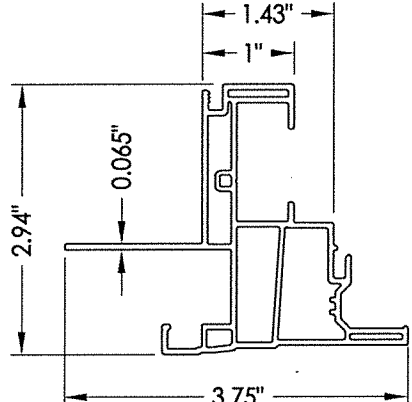
3 FRAME JAMB
