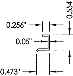
12 JAMB CLIP
